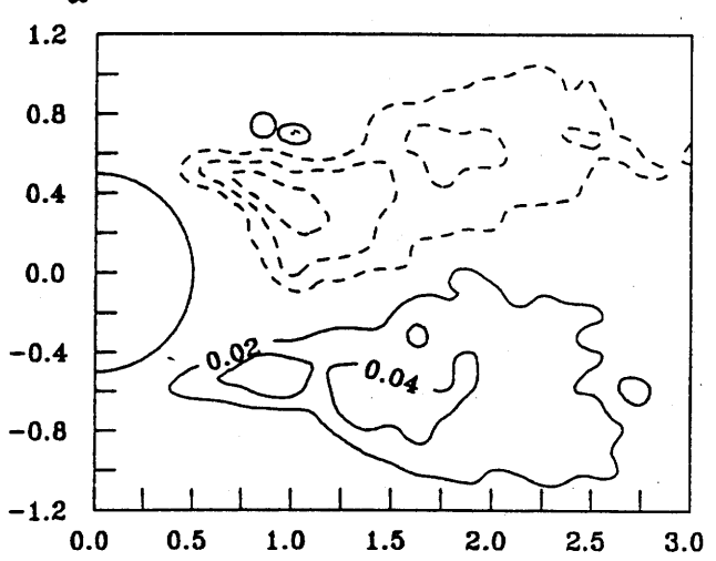
\overline{u'v'} / U_\infty^2
